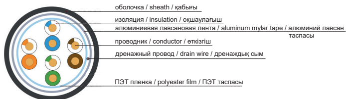
Рисунок 4 – Конструкция кабеля типа F/UTP (количество жил 4×2) / Figure 4 – Cable design of F/UTP type (number of cores 4×2) / Сурет 4 – F/UTP типті кабель дизайны (4×2 талсымдар саны)
