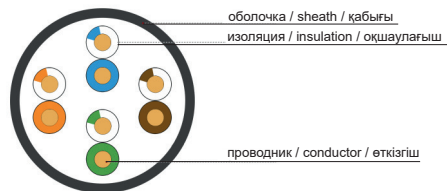
Рисунок 2 – Конструкция кабеля типа U/UTP (количество жил 4×2) / Figure 2 – Cable design of U/UTP type (number of cores 4×2) / Сурет 2 – U/UTP типті кабель дизайны (4×2 талсымдар саны)
