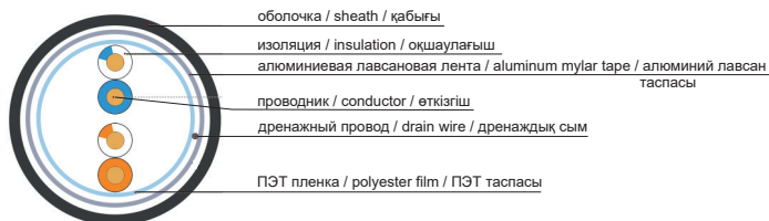
Рисунок 3 – Конструкция кабеля типа F/UTP (количество жил 2×2) / Figure 3 – Cable design of F/UTP type (number of cores 2×2) / Сурет 3 – F/UTP типті кабель дизайны (2×2 талсымдар саны)
