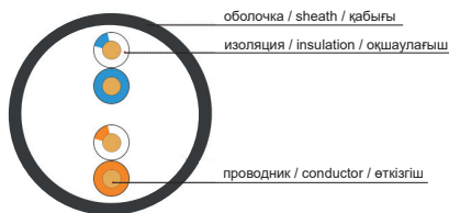
Рисунок 1 – Конструкция кабеля типа U/UTP (количество жил 2×2) / Figure 1 – Cable design of U/UTP type (number of cores 2×2) / Сурет 1 – U/UTP типті кабель дизайны (2×2 талсымдар саны)
