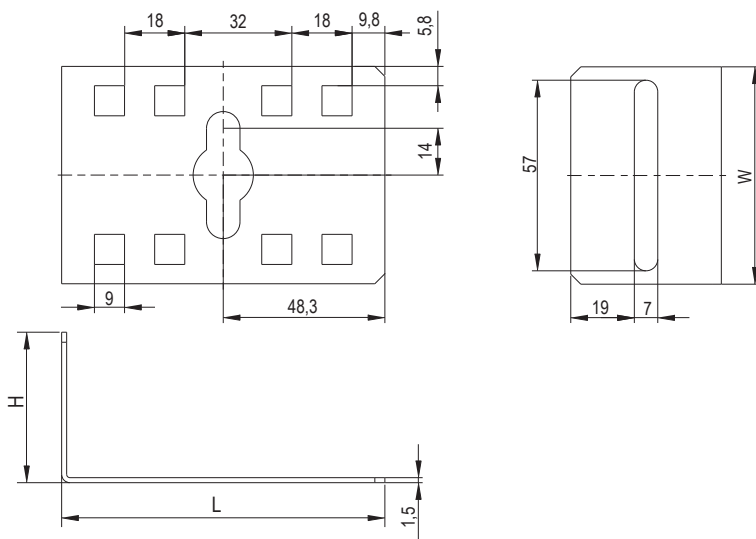
Рисунок / Figure / Сурет 3 – Кронштейн крепления между профилем и дверью / Mounting bracket between profile and door / Профиль мен есік арасындағы бекіту кронштейні (LN00-KRVP-A)
