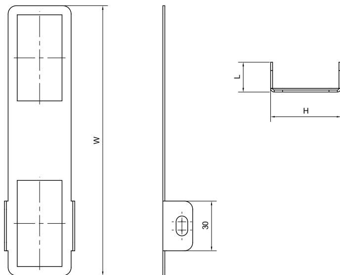
Рисунок / Figure / Сурет 7 – Накладка на ручку под опломбировку / Handle cover plate for sealing / Пломбалауға арналған тұтқаның жапсырмасы
