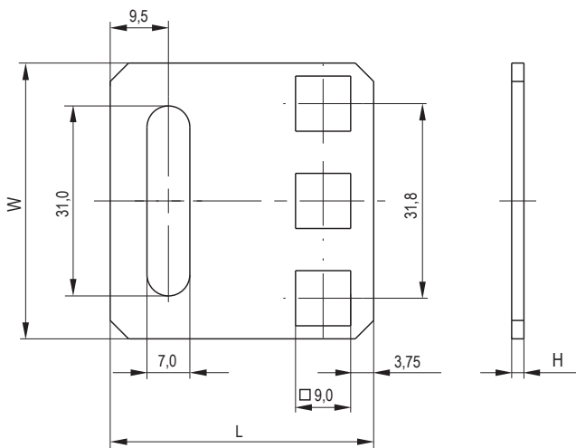
Рисунок / Figure / Сурет 1 – Переходник / Adapter / Жалғастырғыш
