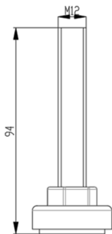
Рисунок / Figure / Сурет 6 – Регулируемая опора (ножка) / Adjustable support (foot) / Реттелетін тірек (аяқ)
