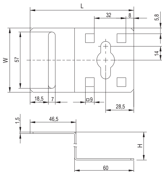
Рисунок / Figure / Сурет 4 – Кронштейн крепления между профилем и боковой стенкой / Mounting bracket between the profile and the side wall / Профиль мен бүйір қабырға арасындағы бекіту кронштейні (LN00-KRVP-B)
