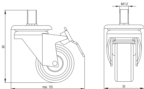
Рисунок / Figure / Сурет 9 – Ролик с тормозом (M12) / Brake roller (M12) / Тежегіш ролик (M12)
