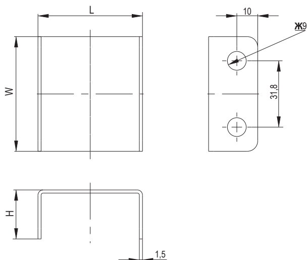
Рисунок / Figure / Сурет 5 – Комплект соединительный для шкафа / Connecting unit for the cabinet / Шкафқа арналған жалғау жиынтығы (ITK-HP-20)
