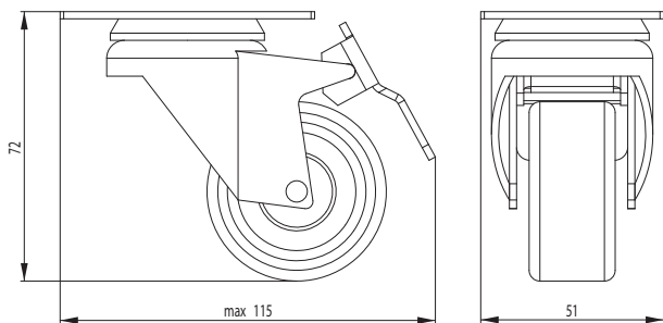
Рисунок / Figure / Сурет 8 – Ролик с тормозом / Brake roller / Тежегіш ролик
