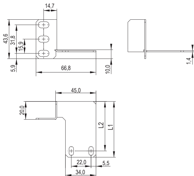
Рисунок / Figure / Сурет 2 – Кронштейн 19" для крепления выключателя / 19" bracket for switch mounting / Ажыратқышты бекітуге арналған 19" кронштейн (LN35-KRKV-G, LN05-KRKV-G, LN35-KRKV-M, LN05-KRKV-M, LN35-KRKV-P, LN05-KRKV-P)
