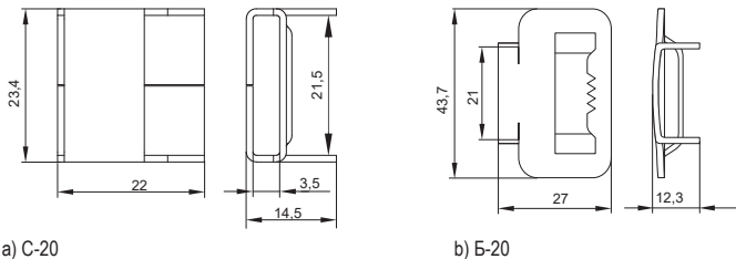
Рисунок / Figure / Сурет 1 – Габаритные размеры скрепы и бугеля / Overall dimensions of the fastener and buckle / Ұстатқыш пен бугелдің габариттік өлшемдер
