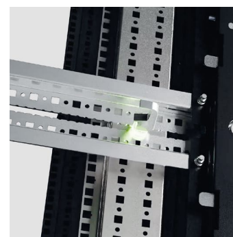
Быстросъемные фиксаторы 19" профиля
