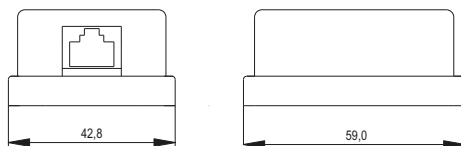
Рисунок / Figure 1 – Розетка / Jacks CS2-3C03U-12-G
