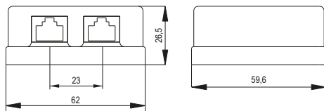
Рисунок / Figure 3 – Розетки / Jacks CS2-1C5EU-22-G, CS2-1C5EF-22-G
