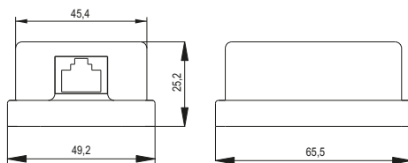
Рисунок / Figure 2 – Розетки / Jacks CS2-1C5EU-12-G, CS2-1C5EF-12-G
