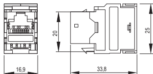
Рисунок / Figure 7 – Модули / Modules CS1-1C6AS-T2-90
