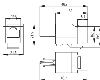
Рисунок / Figure 1 – Модули / Modules CS1-1C5EF-11, CS1-1C06F-11
