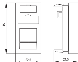
Рисунок / Figure 9 – Вставка / Insert CS6-11M
