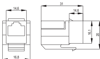
Рисунок / Figure 3 – Модули / Modules CS1-1C5EU-11, CS1-1C06U-11, CS1-1C6AU-11
