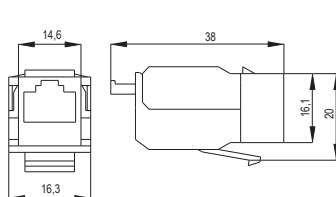
Рисунок / Figure 4 – Модули / Modules CS1-1C5EU-T2, CS1-1C06U-T2, CS1-1C6AU-T2
