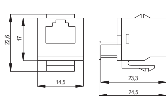
Рисунок / Figure 5 – Модули / Modules CS1-3C03U-12
