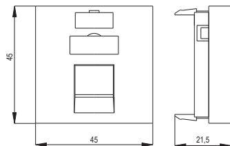
Рисунок / Figure 11 – Вставка / Insert CS6-12M
