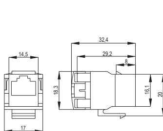
Рисунок / Figure 2 – Модули / Modules CS1-1C5EU-12, CS1-1C06U-12
