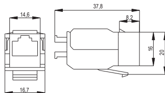
Рисунок / Figure 6 – Модули / Modules CS1-1C5ES-T2, CS1-1C06S-T2, CS1-1C6AS-T2, CS1-1C06S-T2-D, CS1-1C6AS-T2-D
