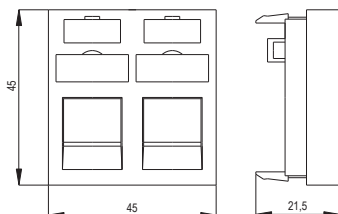
Рисунок / Figure 10 – Вставка / Insert CS6-22M
