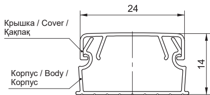
Рисунок 2 – Размеры кабель-канала 24×14 мм / Figure 2 – Dimensions of the cable trunking 24×14 mm / 2 сурет – 24×14 мм кабель-арнаның өлшемдері
