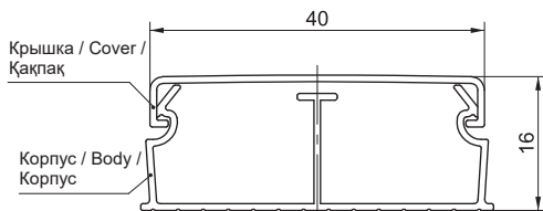
Рисунок 3 – Размеры кабель-канала 40/2×16 мм / Figure 3 – Dimensions of the cable trunking 40/2×16 mm / 3 сурет – 40/2×16 мм кабель-арнаның өлшемдері
