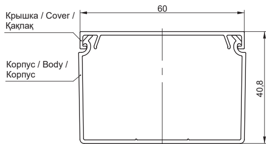
Рисунок 4 – Размеры кабель-канала 60×40 мм / Figure 4 – Dimensions of the cable trunking 60×40 mm / 4 сурет – 60×40 мм кабель-арнаның өлшемдері
