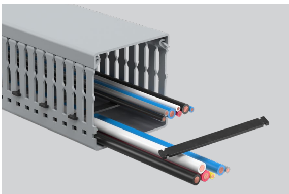
Перфорация под разделители и стяжку внизу боковой стенки для разделения и фиксации провода внутри
