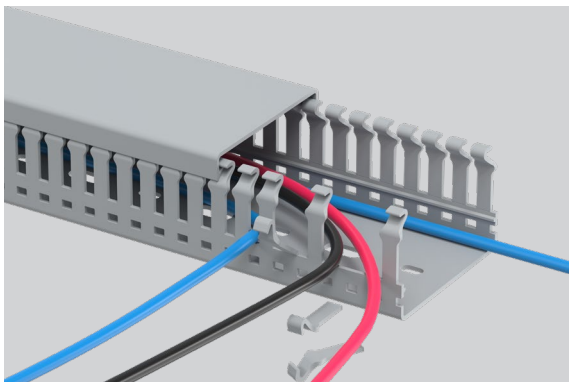
Насечки для удаления зубцов без острых краев/заусенцев
