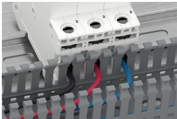
Перфорация шаг перфорации совпадает с шагом вывода контактов автоматических выключателей
